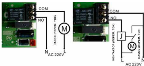
РИСУНОК 3-7 ЭЛЕКТРИЧЕСКОЕ ПОДКЛЮЧЕНИЕ ПОДКАЧИВАЮЩЕГО НАСОСА НА ВХОДЕ НАПРЯМУЮ
