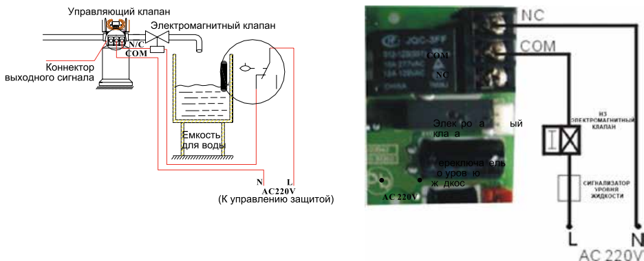
Рисунок 3-1 Электрическое подключение электромагнитного клапана на выпускном трубопроводе
