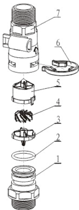
5447020 Расходомер
